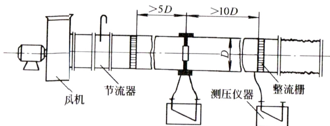
图 A.2.6-3 负压风管式漏风量测试装置
