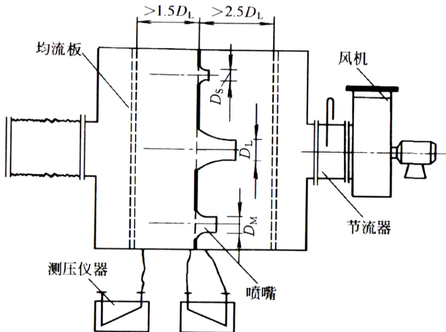
图 A.2.7-4 负压风室式漏风量测试装置
