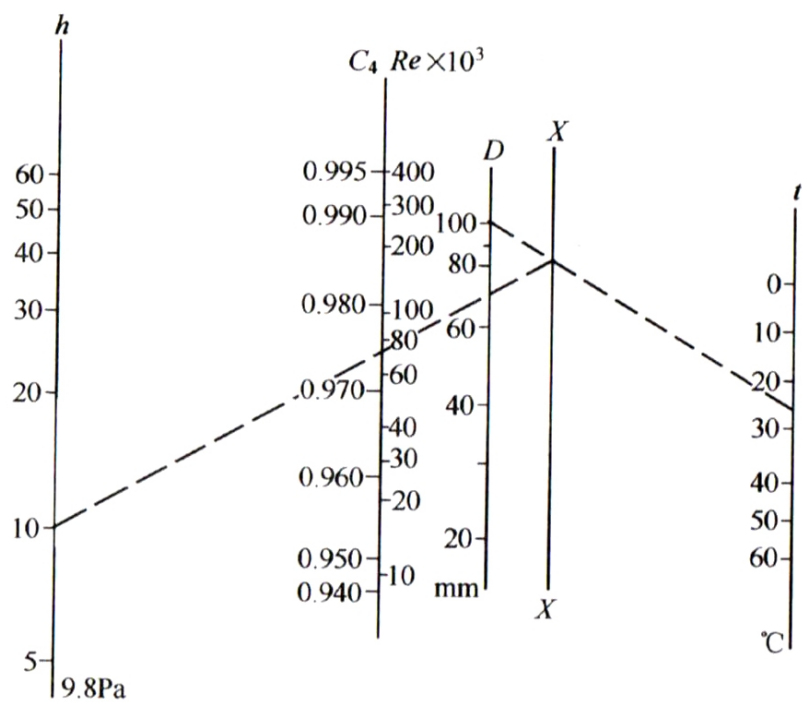
图 A.2.7-3 喷嘴流量系数推算图
