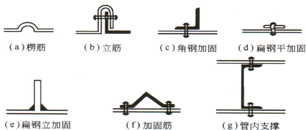
图 4.3.4 风管的加固形式
