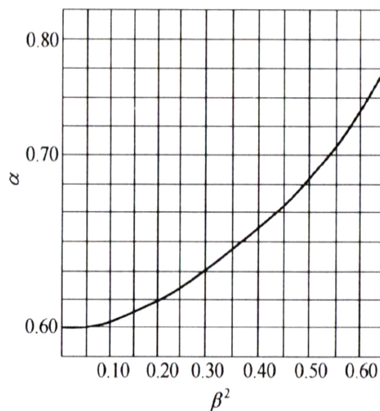
图 A.2.6-2 孔板流量系数图
